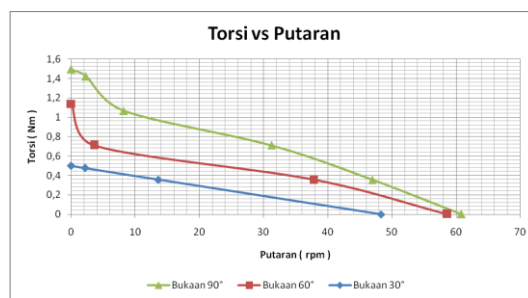
Gambar 4.8 Grafik Putaran vs Torsi menggunakan sudu 1 pada bukaan 30°, 60° dan 90° saluran buang 7 cm dengan ketinggian 0,1 cm.
