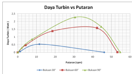
Gambar 4.6 Grafik Putaran Turbin vs Daya Turbin menggunakan sudu 1 pada bukaan 30°, 60° dan 90° saluran buang 6 cm dengan ketinggian 0,1 cm.
