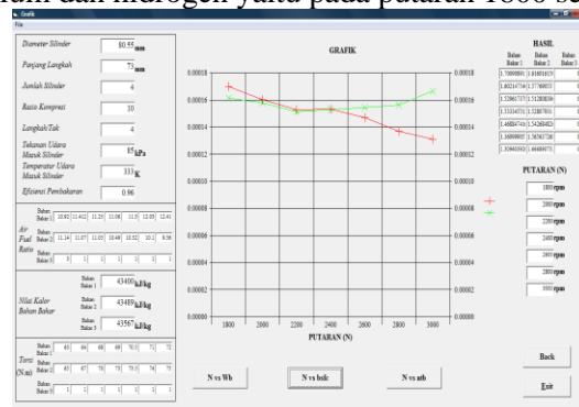
Gambar 3.6 Grafik Putaran vs bsfc
