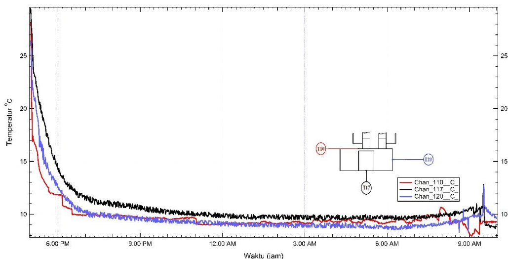
Gambar 8 Grafik Temperatur vs Waktu Adsorpsi Metanol pada Gelas Ukur
