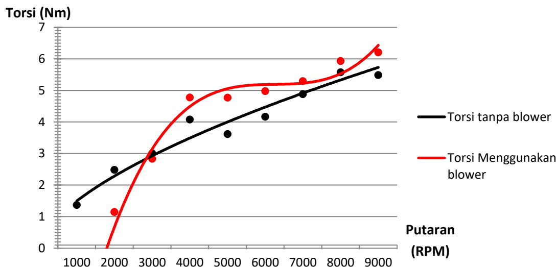
Gambar 3 Perbandingan Grafik Torsi Vs Putarant an pada saat menggunakan blower
