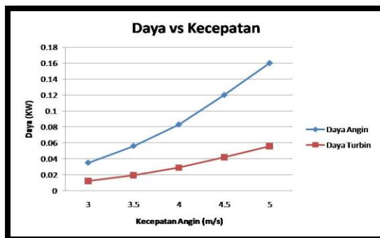
Gambar 6 Grafik perbandingan daya dengan kecepatan angin
