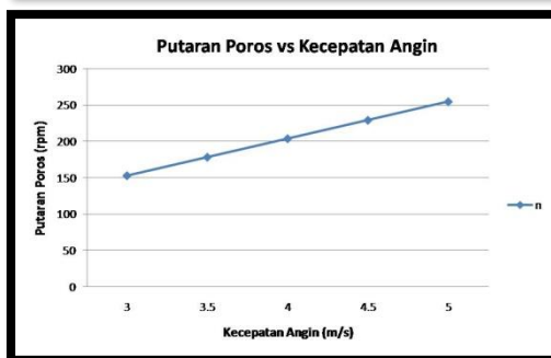
Gambar 7 Grafik Putaran poros vs kecepatan angin
