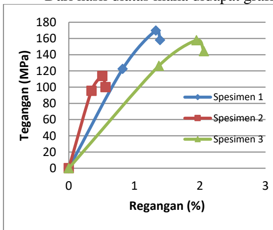
Gambar 3. Grafik Tegangan vs Regangan sudut kampuh 45°.
