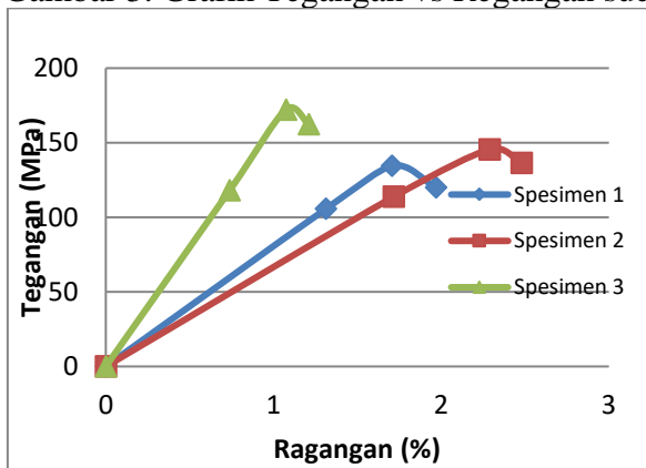
Gambar 4. Grafik tegangan vs regangan sudut kampuh 55°
