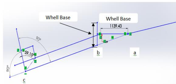
Gambar 4.6 Pemeriksaan sudut overturn .
