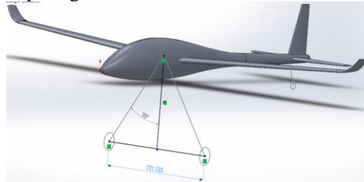
Gambar 4.5 Posisi sudut overturn dengan kemiringan 35°.
