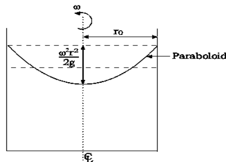
Gambar 2.1 Teh Cangkir yang di aduk adalah sebuah Aplikasi Vorteks paksa [2]
