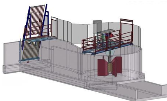
Gambar 2.3 Turbin vorteks
