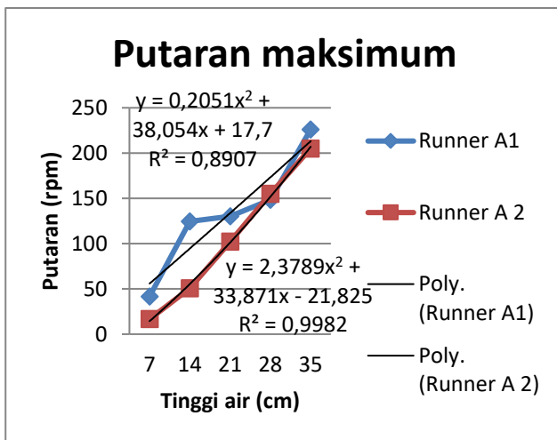
Gambar 4.1 Grafik putaran tanpa beban
