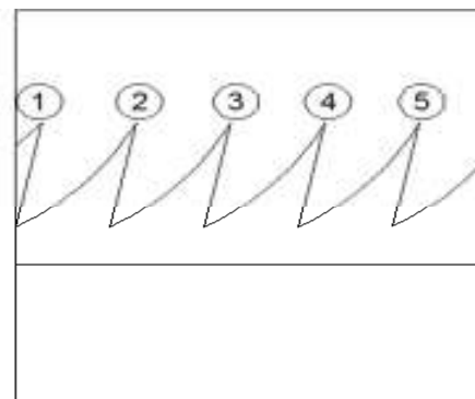
Gambar 4. Cara Penghitungan Jumlah Mata Gergaji ( n_p )
