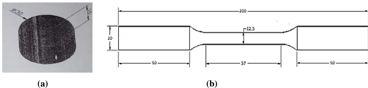
Gambar 2.1 Uji kekerasan ASTM E10 (a), Uji Tarik ASTM E8 (b) [4]
