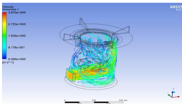
Gambar 4 Hasil Simulasi Kecepatan Udara pada Kompur
