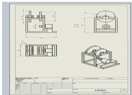
Gambar 9. Gambar teknik alat pemotong singkong
