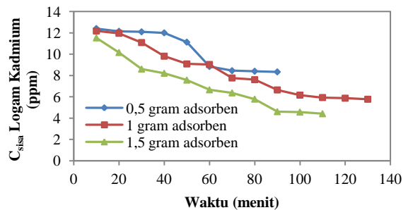
Gambar 1. Hubungan C sisa Ion Logam Kadmium terhadap Waktu
