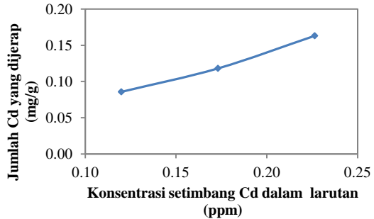
Gambar 3. Pola Isotherm Adsorpsi Cangkang Telur Bebek terhadap Ion Logam Kadmium
