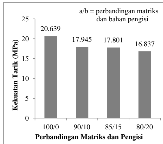
Gambar 1. Pengaruh Kandungan Bahan Pengisi Terhadap Kekuatan Tarik Komposit Polipropilena
