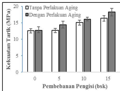
Gambar 2. Kekuatan Tarik ( Tensile strength ) Film Lateks Karet Alam Bepengisi Nanokristalin Selulosa dan Penyerasi Alkanolamida
