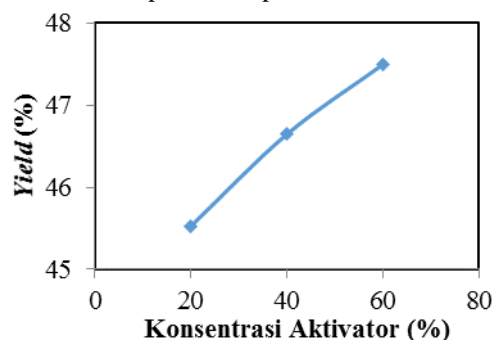
Gambar 1. Pengaruh Konsentrasi Aktivator terhadap Yield Karbon Aktif
