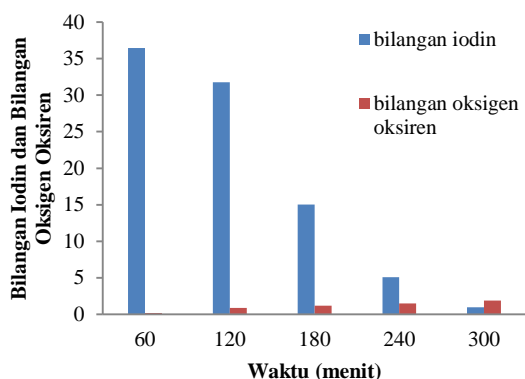
Gambar 6. Hubungan antara Bilangan Iodin dan Bilangan Oksigen Oksiren
