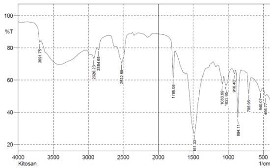
Gambar 1. Analisa FT-IR
