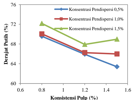
Gambar 2. Pengaruh Konsistensi Pulp terhadap Derajat Putih Kertas pada Kondisi Suhu Flotasi 50 °C dan Waktu Flotasi 40 menit
