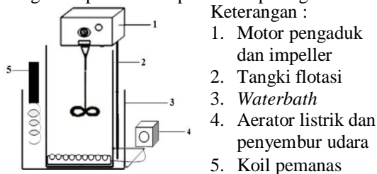
Gambar 1. Rangkaian Peralatan Flotasi
