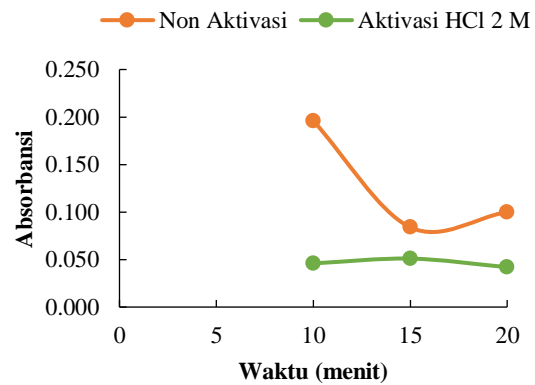
Gambar 7. Grafik hubungan waktu kontak dengan absorbansi pada dosis adsorben 0,1 g
