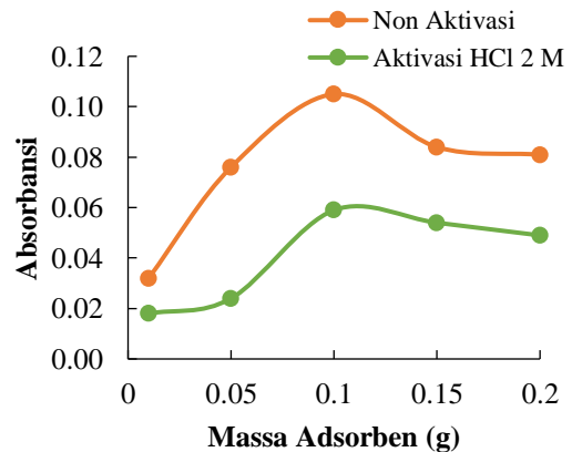
Gambar 5. Grafik hubungan massa adsorben dengan absorbansi
